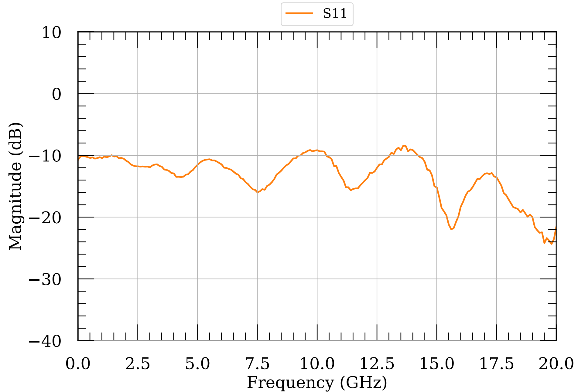
LNA S-params module005v2
